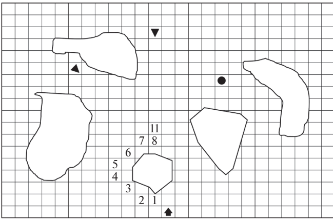
Рис. 4. Поле боя для алгоритма 1
