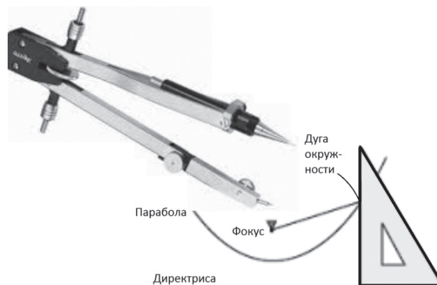
Рис. 1. Построение параболы циркулем и угольником
