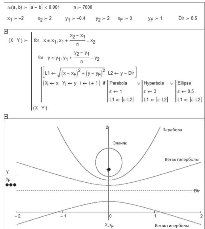
Рис. 4. Построение гиперболы, параболы и эллипса (анимация: https://www.picusercommunity.com/thread/140084 )
