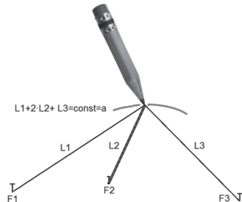
Рис. 6. Рисование эллипса с тремя фокусами
