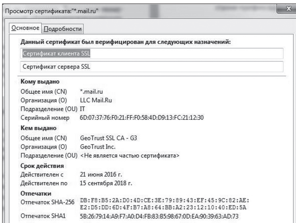
Рис. 5. SSL-сертификат mail.ru
