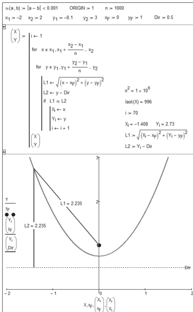
Рис. 2. Построение параболы
