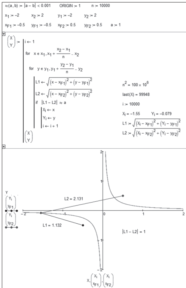
Рис. 3. Построение гиперболы
